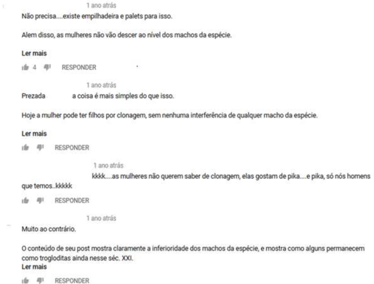
Figura 1 – Comentários diversos
