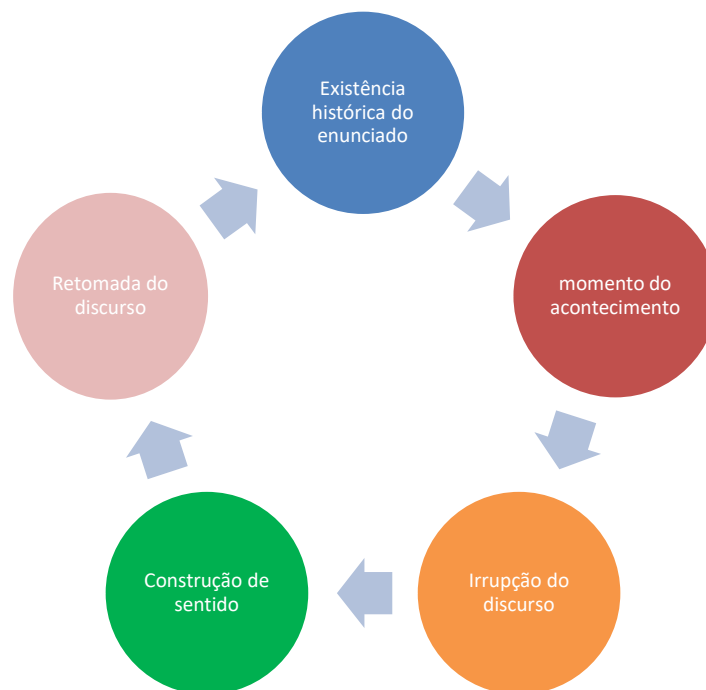
Figura 3 - Relações enunciativas
