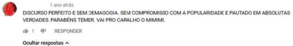
Figura 2 – Comentário 2
